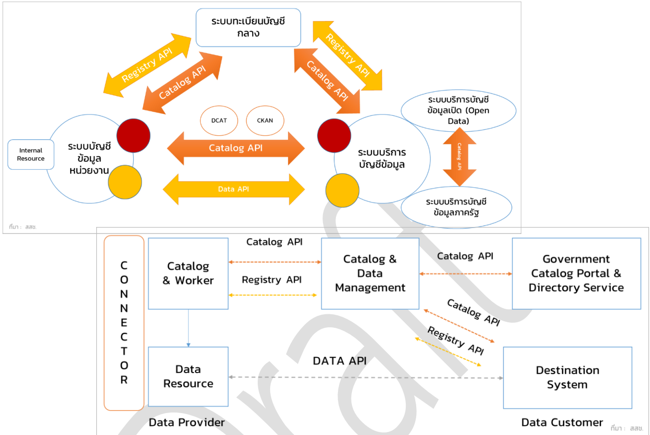
รูปที่: 34 การทำงานระหว่าง API ในระบบบัญชีข้อมูลภาครัฐ
