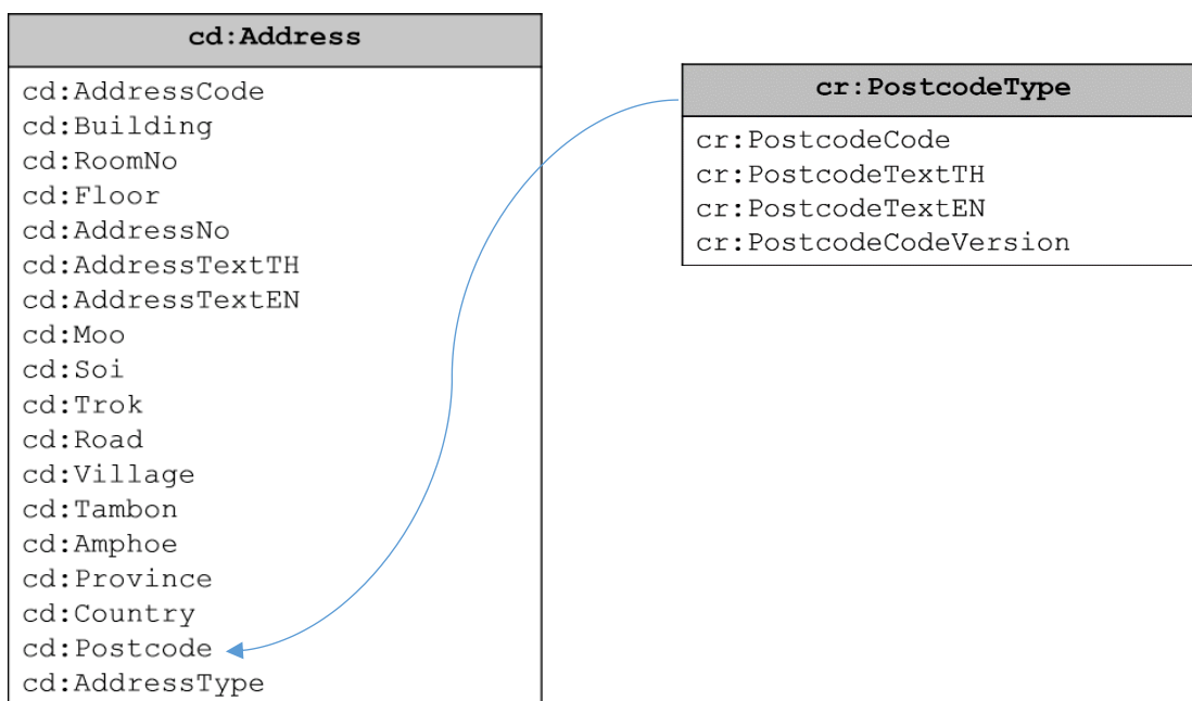
รูปที่ 48 ประเภทข้อมูลที่อ้างอิง
