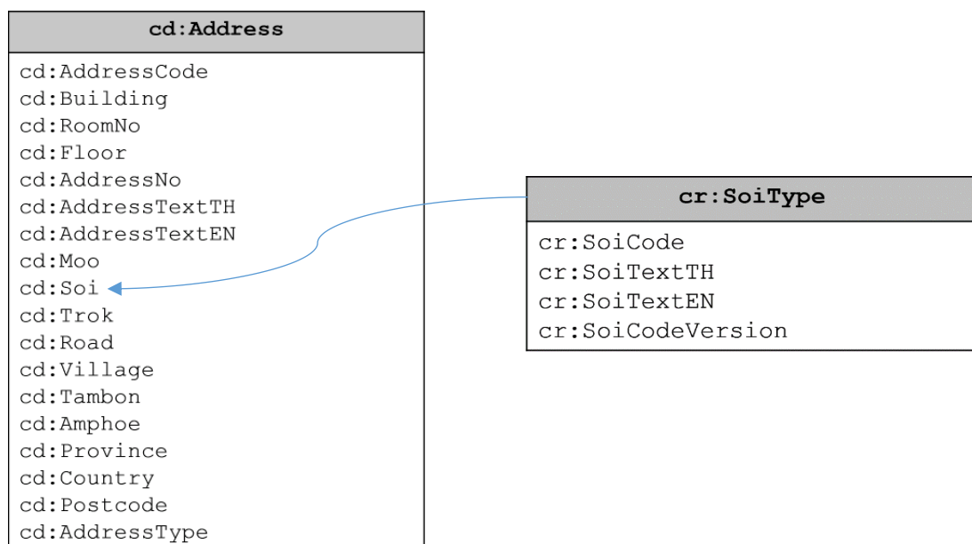
รูปที่ 43 ประเภทข้อมูลย่อย
