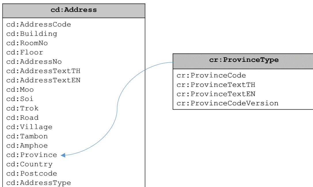
รูปที่ 13 ประเภทข้อมูลจังหวัด
