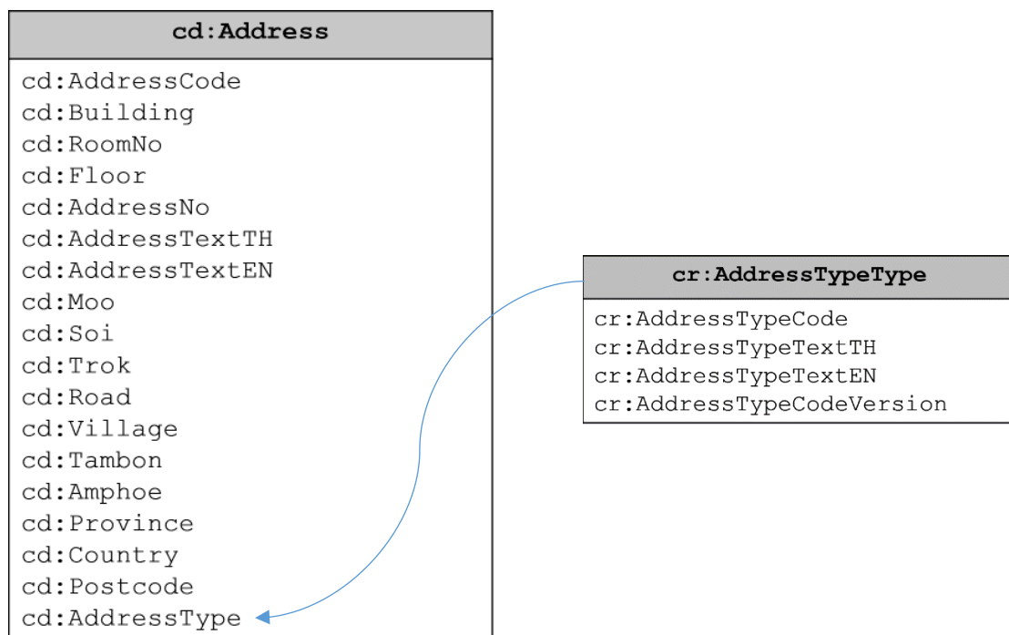
รูปที่ 28 ประเภทข้อมูลประเภทที่อยู่
