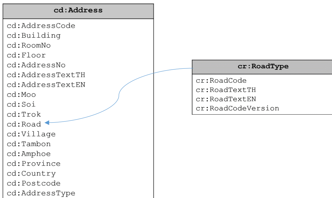
รูปที่ 33 ประเภทข้อมูลถนน
