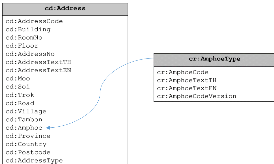
รูปที่ 18 ประเภทข้อมูลอำเภอ
