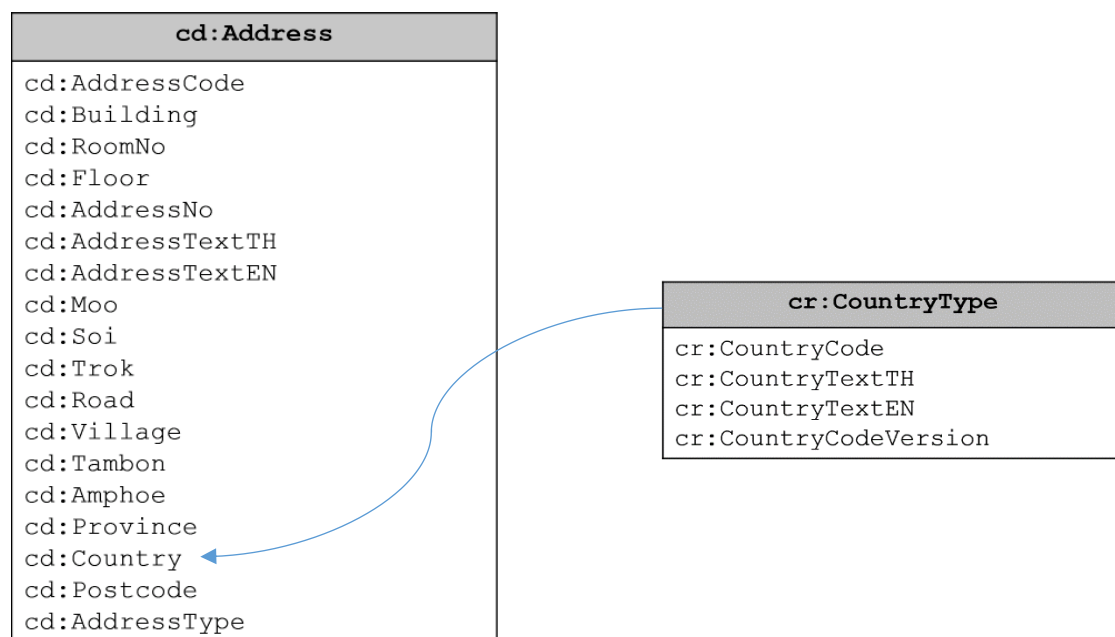
รูปที่ 8 ประเภทข้อมูลประเทศ
