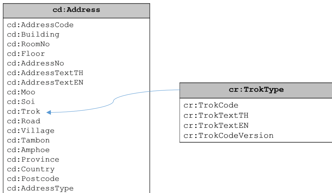
รูปที่ 38 ประเภทข้อมูลตรอก
